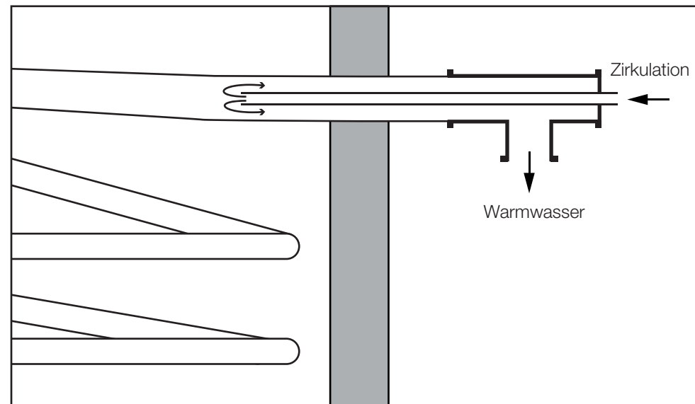
Funktionsschema der Zirkulationslanze
