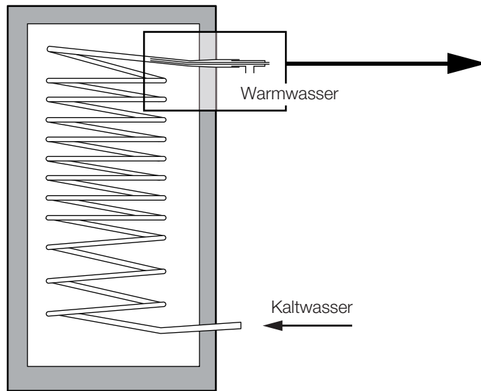
Hygienespeicher mit Zirkulationslanze
